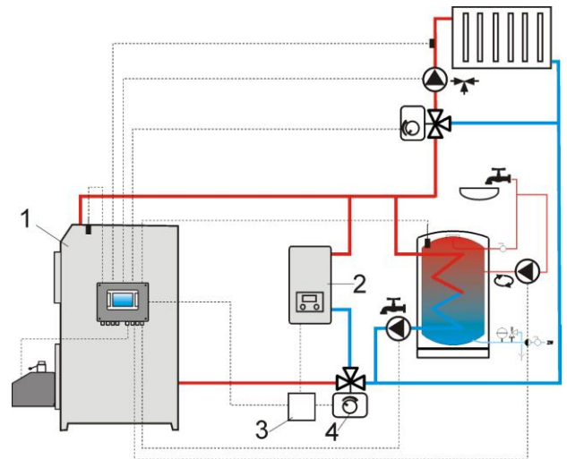
Schemat hydrauliczny z kotłem rezerwowym w obiegu zamkniętym, gdzie: 1 – regulator, 2 – kocioł rezerwowo, 3 – przekaźnik, 4 – zawór przełączający (z wyłącznikami krańcowymi).
