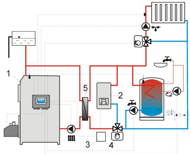
Schemat hydrauliczny z kotłem rezerwowym w obiegu otwarcie-zamkniętym, gdzie: 1 – regulator, 2 – kocioł rezerwowo, 3 – przekaźnik, 4 – zawór przełączający (z wyłącznikami krańcowymi), 5 – wymiennik ciepła, zalecane ustawienie: priorytet CWU = wyłączony, wymiennik ciepła = TAK.
