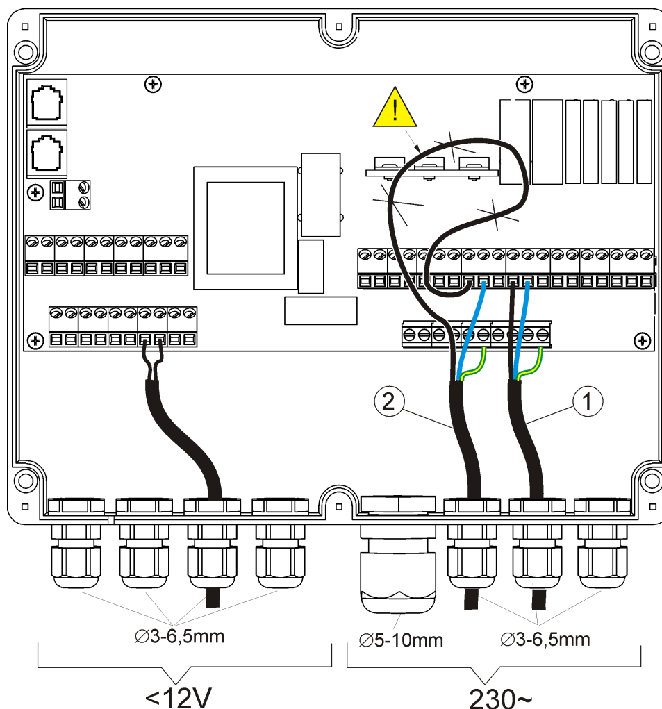
Rys. 21 Podłączenie przewodów, gdzie 1 – przewód podłączony poprawnie, 2 - przewód podłączony błędnie (nie dopuszcza się zwijania nadmiaru przewodów wewnątrz urządzenia).
