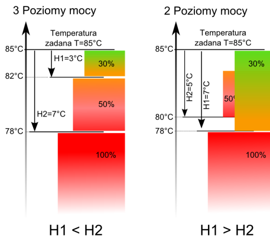
Rys. 8 Histerezy H1 i H2 modulacji mocy
