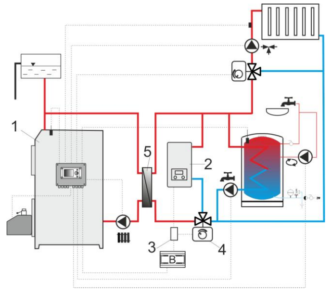
Rys. 26 7 Schemat hydrauliczny z kotłem rezerwowym w obiegu otwarto-zamkniętym,
