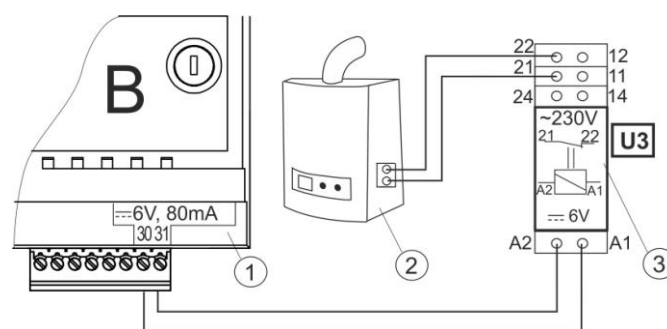
Rys. 24 Przykładowy schemat układu do podłączenia kotła rezerwowego do regulatora, gdzie: 1- moduł B, 2 – kocioł rezerwy (gazowy lub olejowy), 3 –przełącznik RM 84-2012-35-1006 i podstawka GZT80 RELPOL.
