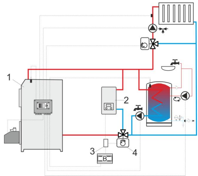
Rys. 25 6 Schemat hydrauliczny z kotłem rezerwowym w obiegu zamkniętym, gdzie: 1 – regulator, 2 – kocioł rezerwowy, 3 – przekaźnik (Rys. 27), 4 – zawór przełączający (z wyłącznikami krańcowymi).
