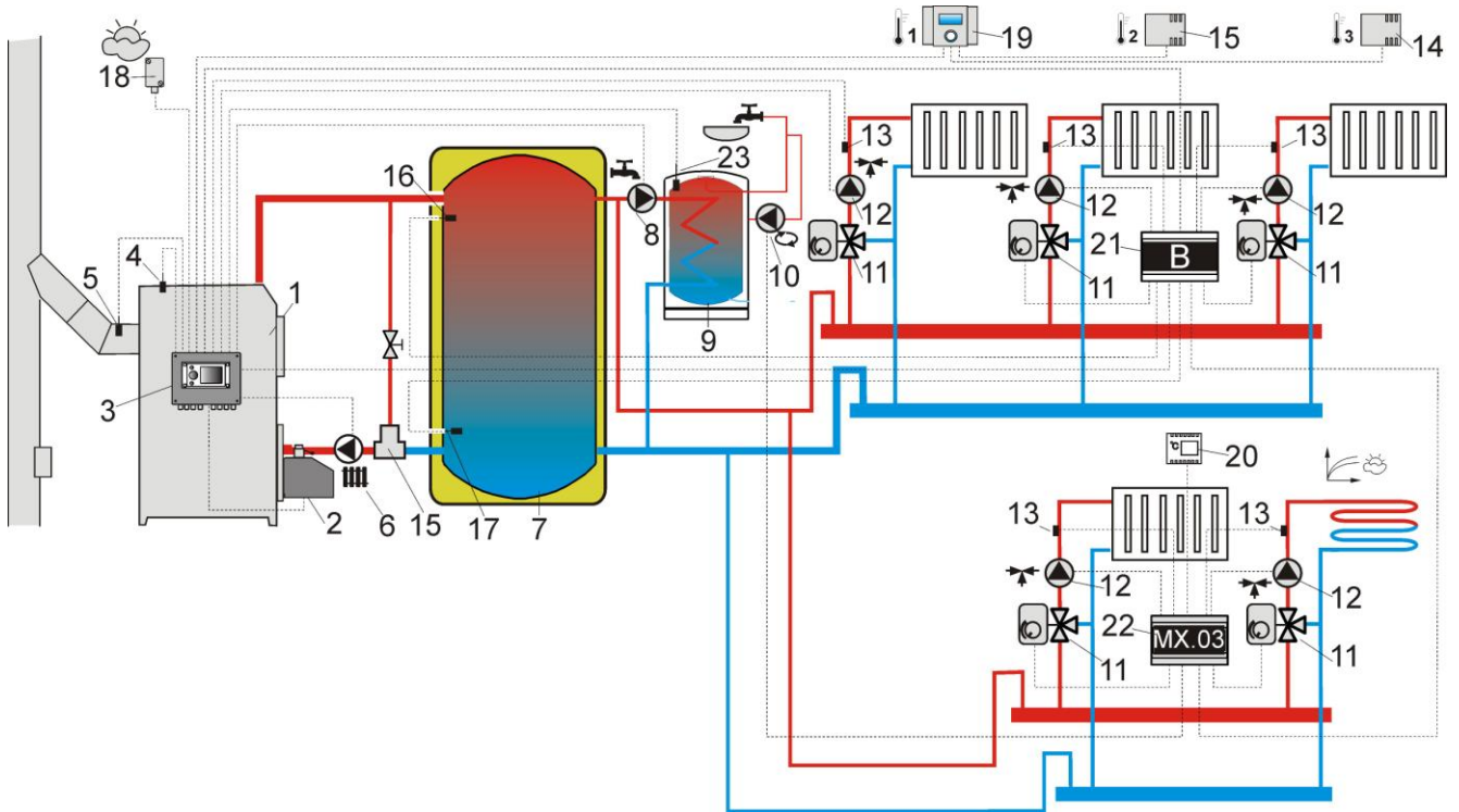
Rys. 19 Schemat z buforem ciepłym oraz z 5 mieszaczymi obiegami grzewczymi 4 , gdzie: 1 – kocioł, 2 – palnik, 3 – regulator, 4 – czujnik temperatury kotła CT4, 5 – czujnik temperatury spalin CT2S, 6 – pompa kotła, 7 – bufor ciepły, 8 – pompa ciepłej wody użytkowej, 9 – zasobnik ciepłej wody użytkowej, 10 – pompa cyrkulacyjna, 11 – zawór trójdrogowy z siłownikiem, 12 – pompa obiegu mieszacza, 13 – czujnik temperatury obiegu mieszacza CT4, 14 – czujnik pokojowy CT7, 15 – czujnik pokojowy CT7, 16 – czujnik górny temperatury bufora CT4, 17 – czujnik dolny temperatury bufora CT4, 18 – pogodowy czujnik temperatury CT4-P, 19 – panel pokojowy ecoSTER200 z funkcją termostatu pokojowego, 20 – standardowy termostat pokojowy (zwierno/rozwierny), 21 – dodatkowy moduł B, 22 – dodatkowy moduł MX.03, 23 – czujnik temperatury ciepłej wody użytkowej.
