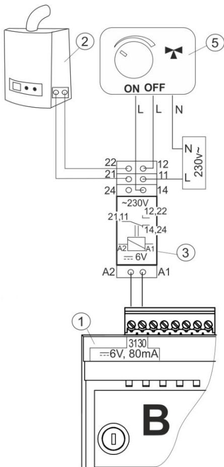
Rys. 27 Schemat elektryczny sterowania zaworem przełączającym kotła rezerwowego, gdzie: 1 – moduł B, 2 – kocioł rezerwowy, 3 – przekaźnik, 5 – siłownik zaworu przełączającego (z wyłącznikami krańcowymi), uwaga: zaciski 22,21,24 muszą być odseparowane galwanicznie od zacisków 12,11,14.
