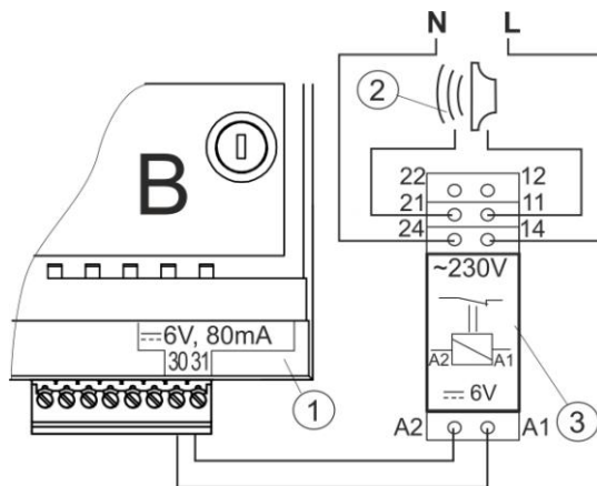
Rys. 28 Podłączenie zewnętrznego urządzenia alarmowego, gdzie: 1- moduł B, 2 -zewnętrzne urządzenie alarmowe, 3 – przekaźnik.
